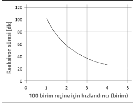
Diagram 2: Hızlandırıcı konsantrasyonuna bağlı olarak 80 °C'de reaksiyon süresi, Gelnorm (CQP021-5 / ISO 9396)
